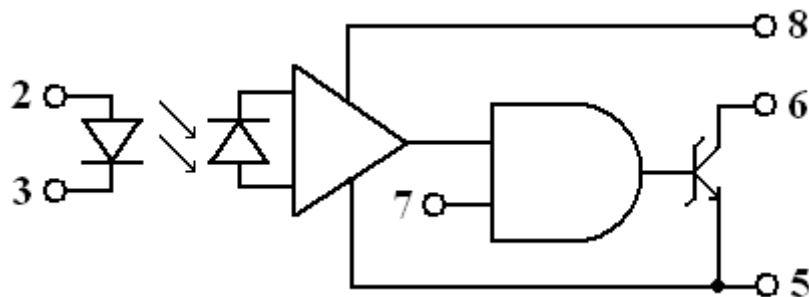
器件原理图
