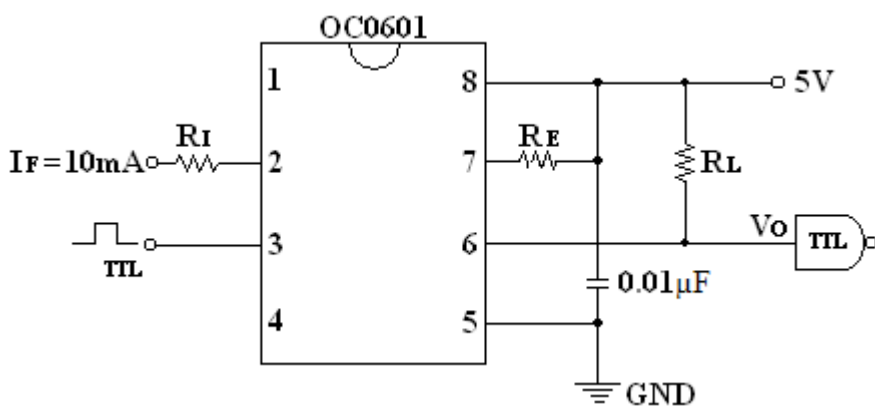
典型应用图
