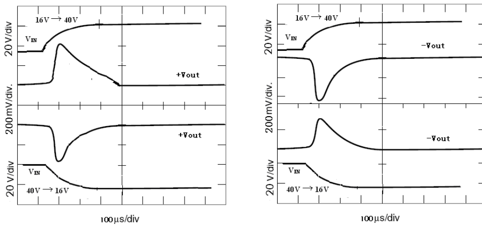
图 14 GTR2815D (F) 输入电压阶跃响应
