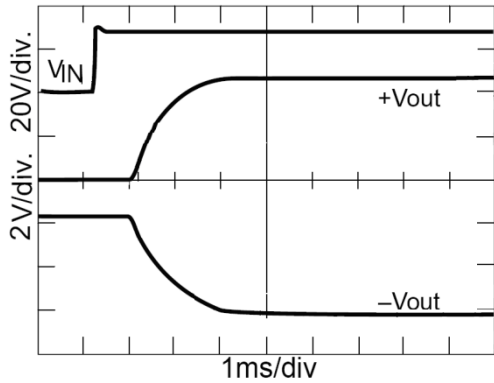
图 6 GTR2805D (F) 启动延时/过冲
