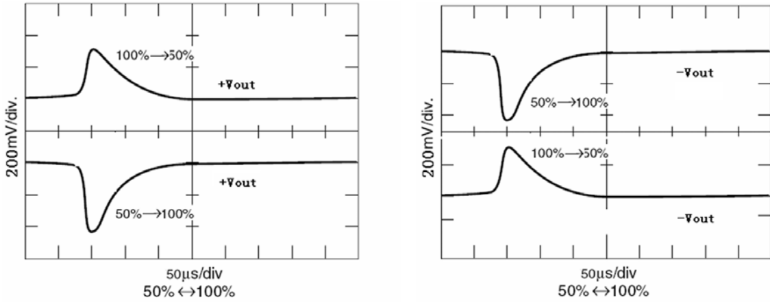
图 9 GTR2805D (F) 负载阶跃响应
