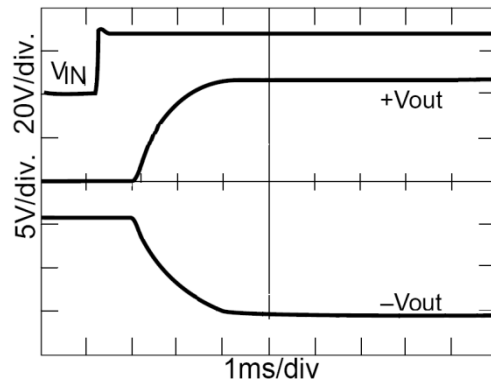
图 7 GTR2812D (F) 启动延时/过冲
