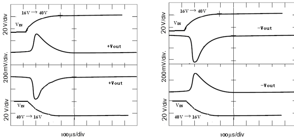
图 13 GTR2812D (F) 输入电压阶跃响应
