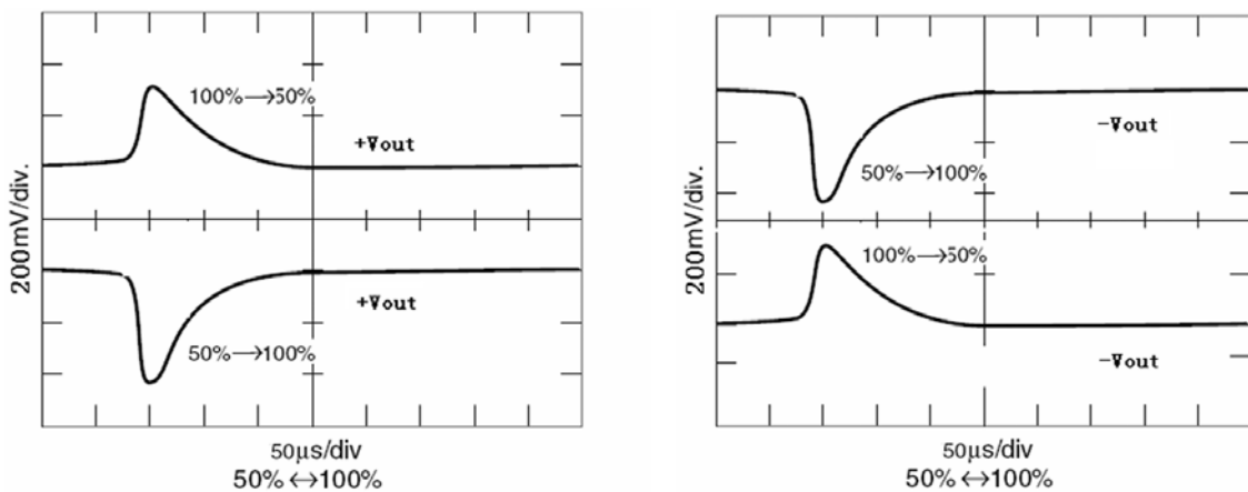
图 11 GTR2815D (F) 负载阶跃响应
