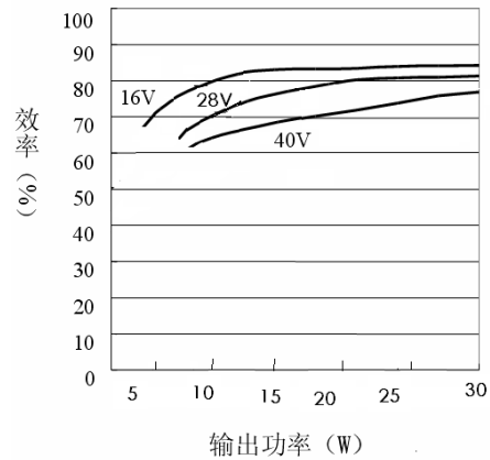
图 19 GTR2812D (F) 效率特性曲线
