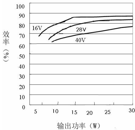
图 20 GTR2815D (F) 效率特性曲线
