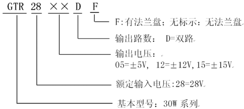
图 3 产品型号示意图
