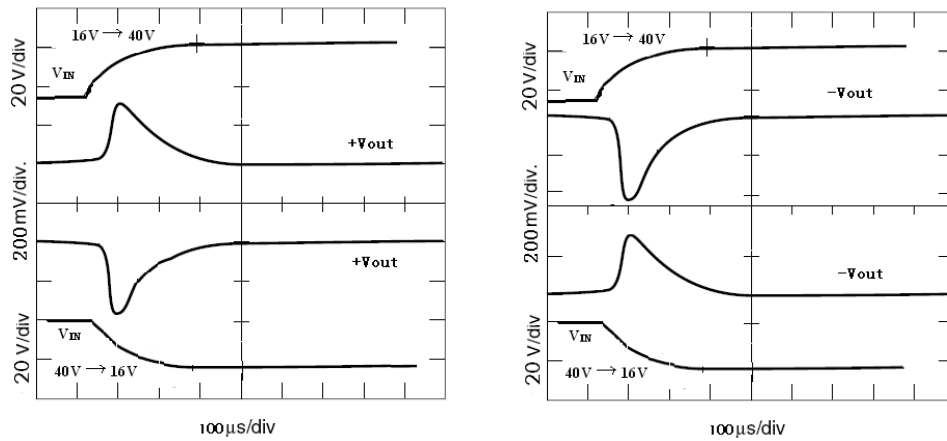
图 12 GTR2805D (F) 输入电压阶跃响应
