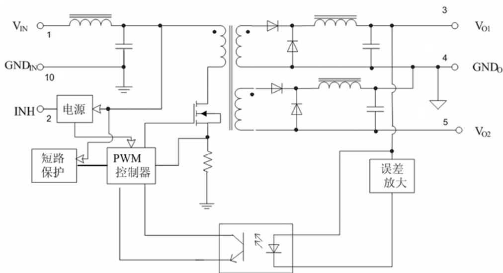
图 1 电原理框图
