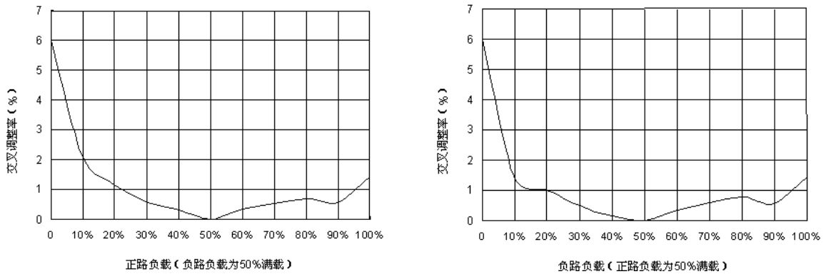
图 16 GTR2812D (F) 交叉调整率波形
