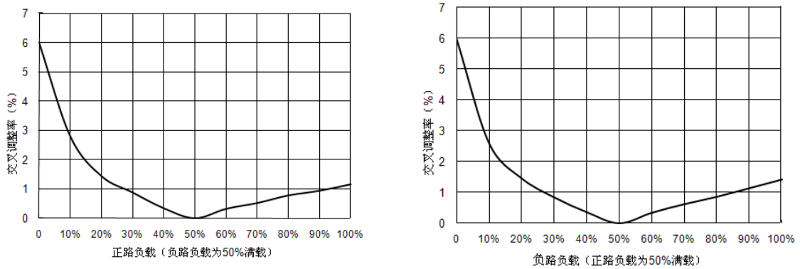
图 15 GTR2805D (F) 交叉调整率波形
