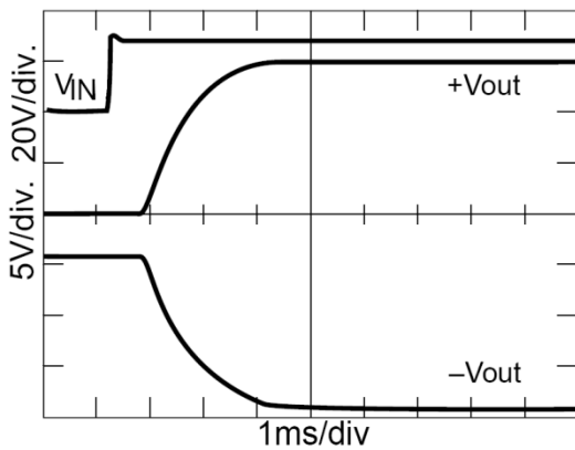
图 8 GTR2815D (F) 启动延时/过冲
