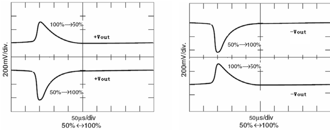
图 10 GTR2812D (F) 负载阶跃响应
