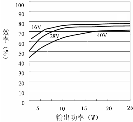
图 18 GTR2805D (F) 效率特性曲线
