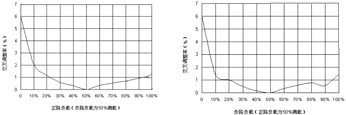
图 17 GTR2815D (F) 交叉调整率波形
