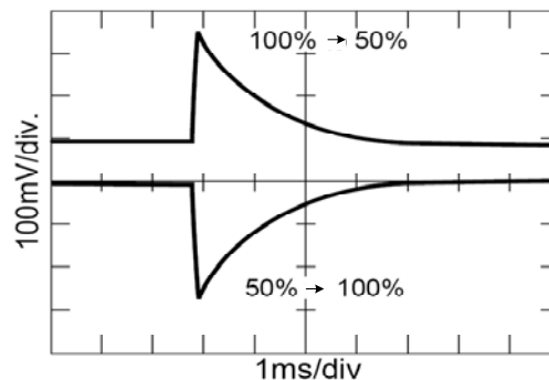
图 9 GFL2828S 负载阶跃响应
