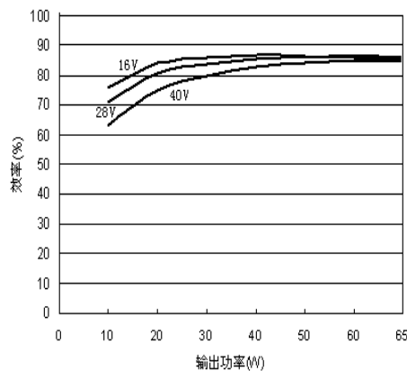
图 13 GFL2828S 效率特性曲线
