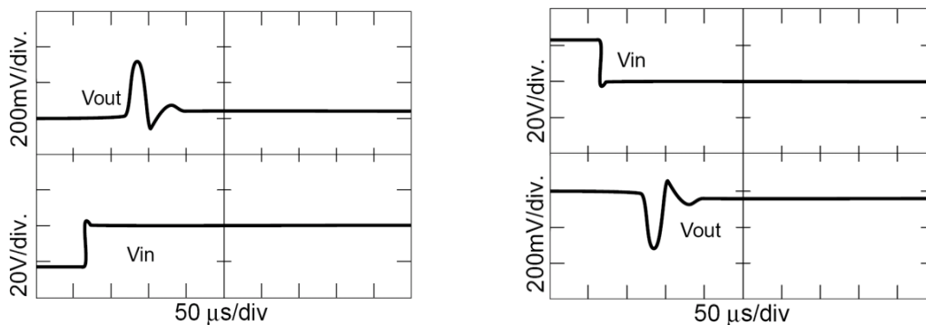
图 11 GFL2828S 输入电压阶跃响应
