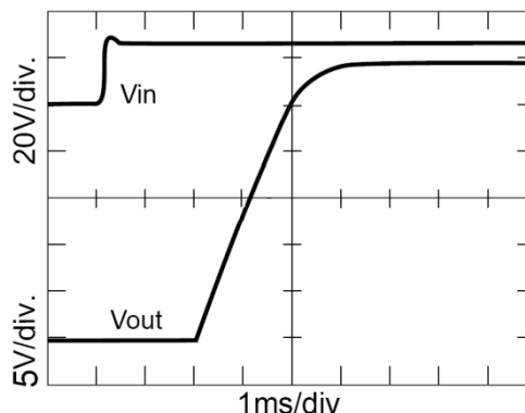
图 7 GFL2828S 启动延时/过冲
