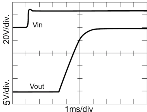
图 6 GFL2825S 启动延时/过冲
