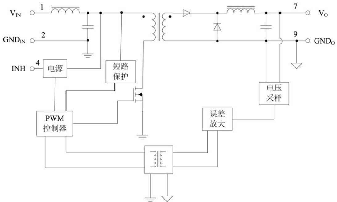
图 1 GFL2825S、GFL2828S 电原理框图
