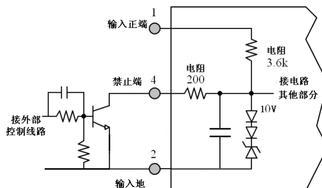
图 5 禁止端连接图
