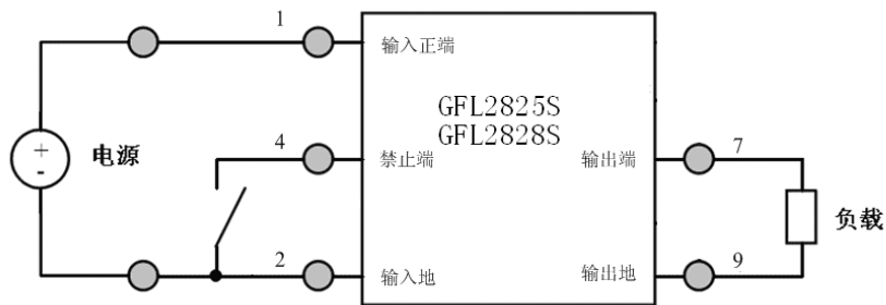
图 4 GFL2825S、GFL2828S 典型应用
