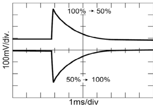
图 8 GFL2825S 负载阶跃响应
