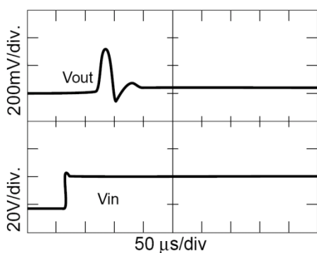
图 10 GFL2825S 输入电压阶跃响应
