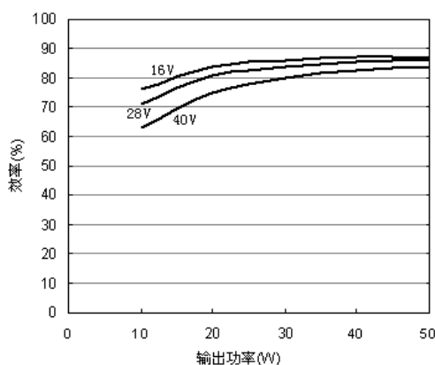
图 12 GFL2825S 效率特性曲线
