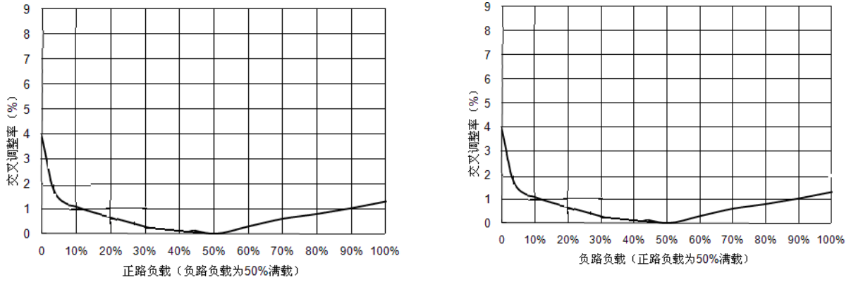
图 16 GFL2812D 交叉调整率波形
