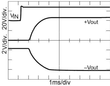
图 6 GFL2805D 启动延时/过冲
