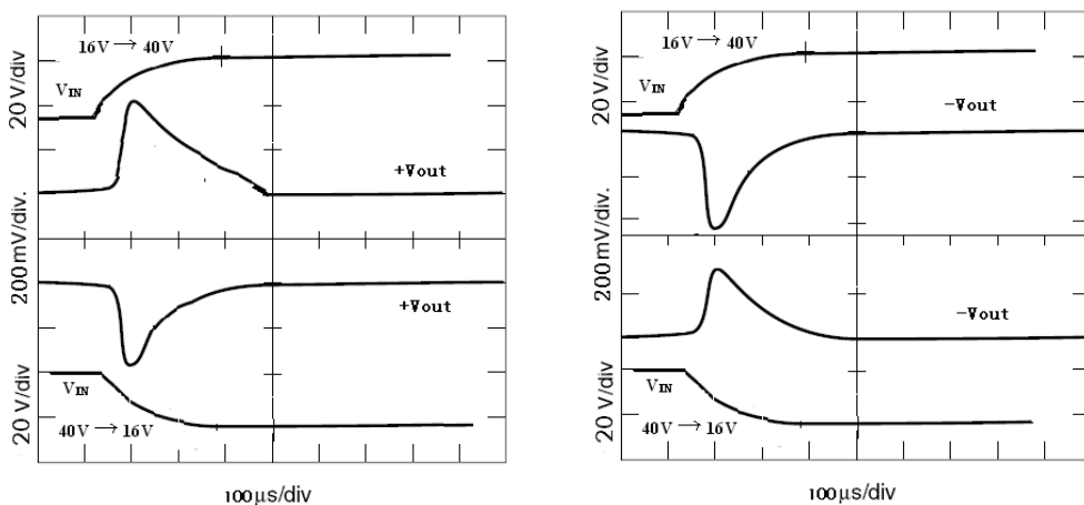
图 14 GFL2815D 输入电压阶跃响应
