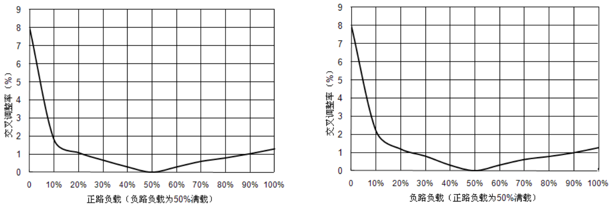
图 15 GFL2805D 交叉调整率波形
