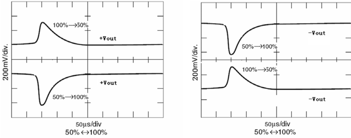
图 10 GFL2812D 负载阶跃响应
