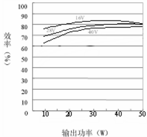
图 19 GFL2812D 效率特性曲线
