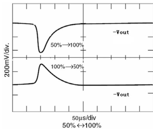
图 9 GFL2805D 负载阶跃响应
