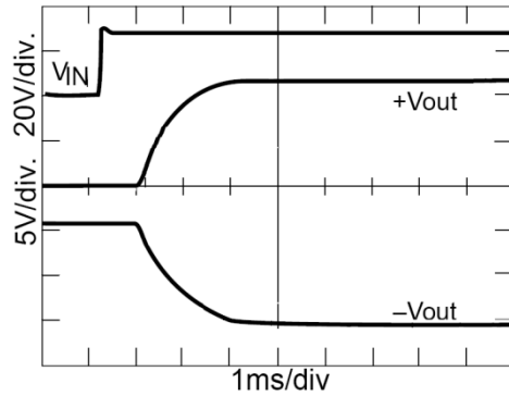
图 7 GFL2812D 启动延时/过冲
