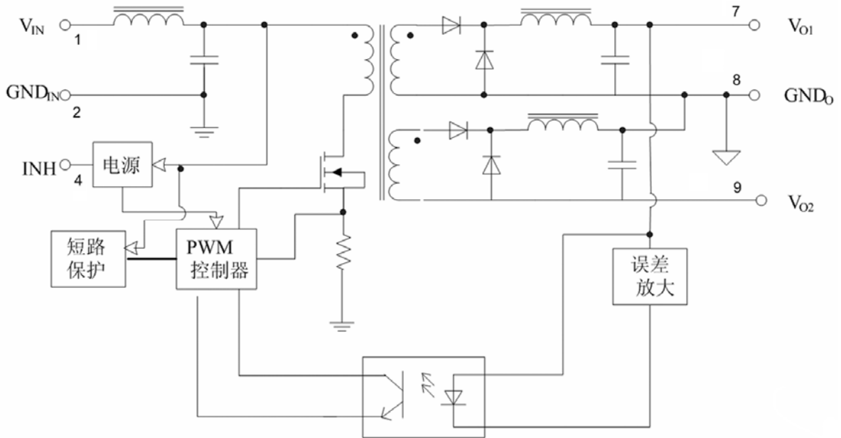
图 1 电原理框图
