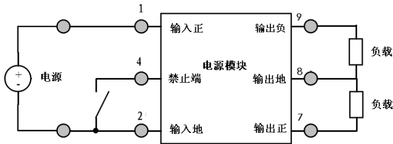
图 4 典型应用
