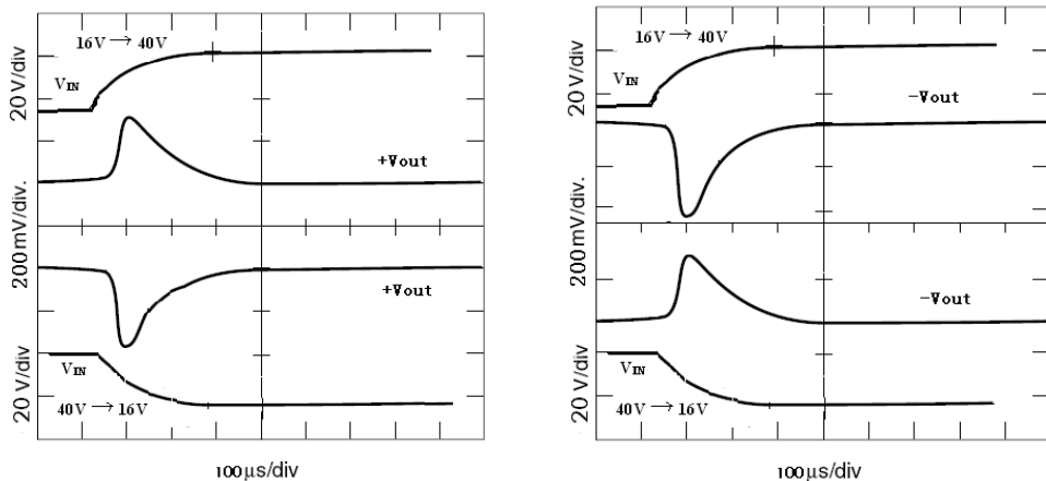
图 13 GFL2812D 输入电压阶跃响应
