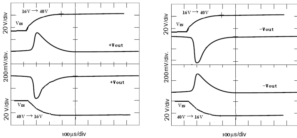
图 12 GFL2805D 输入电压阶跃响应
