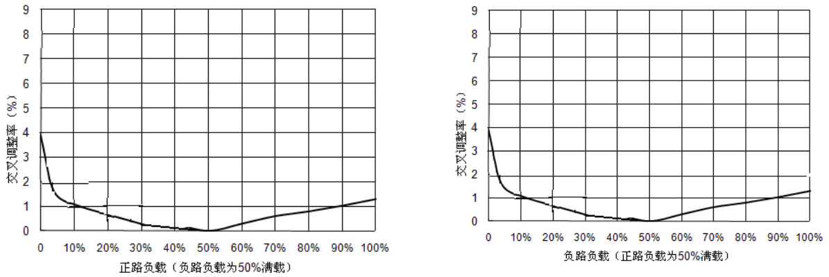
图 17 GFL2815D 交叉调整率波形
