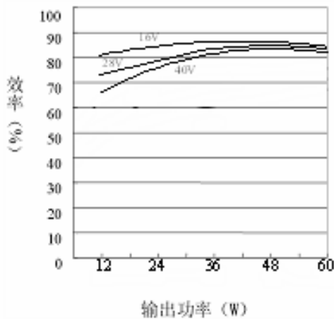
图 18 GFL2805D 效率特性曲线
