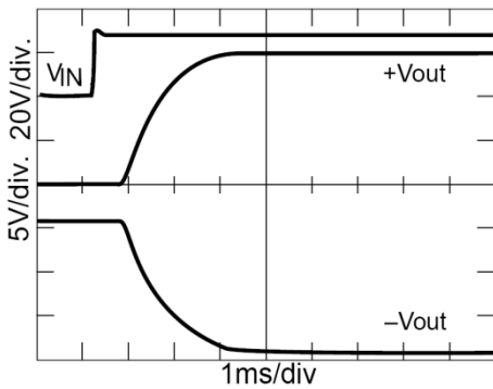
图 8 GFL2815D 启动延时/过冲
