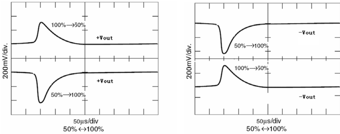
图 11 GFL2815D 负载阶跃响应
