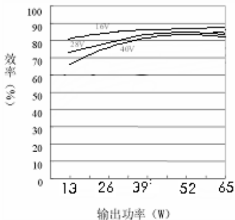
图 20 GFL2815D 效率特性曲线
