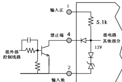
图 5 禁止端连接图
