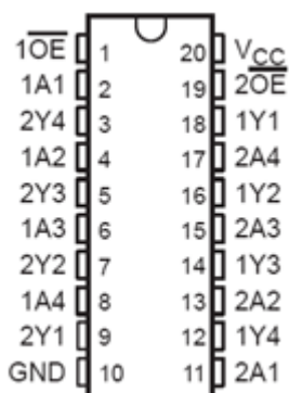
D 型、F 型引出端示意图
